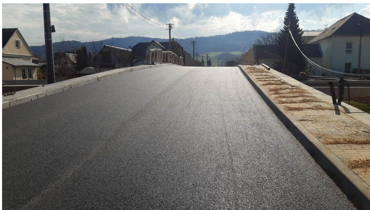
Obrázek 4: finální vrstvy vozovky SO35
